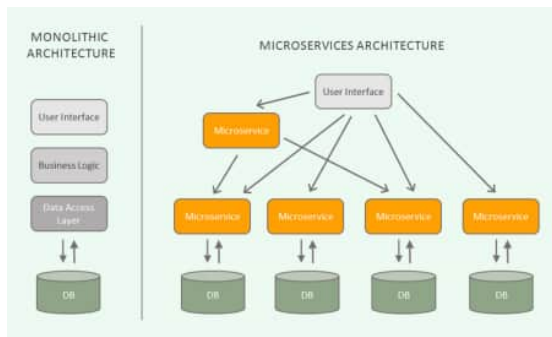
Рис. 2.8 – Схема моноліту та мікросервісної архітектур
