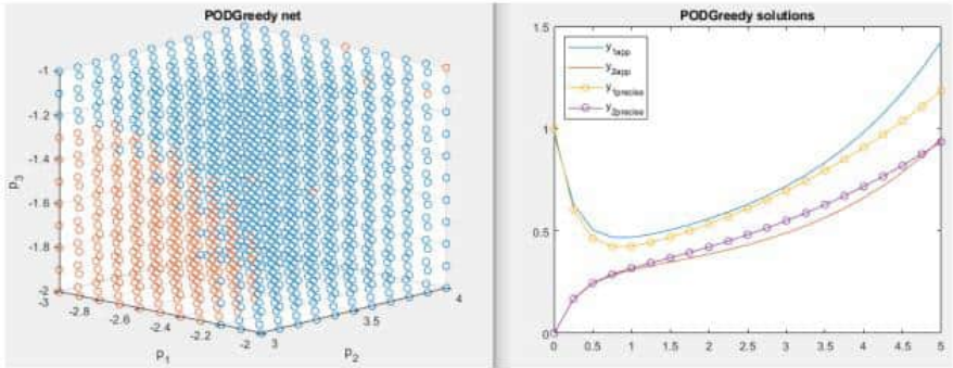
Рис. 4.10 – Графік сітки параметрів і розподілу розв’язків y_1, y_2 прикладу 4.1.4 – точні і наближені (PODGreedy)
